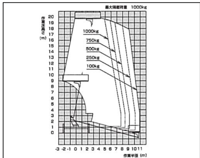
TZ-20A 作業範囲図 アウトリガ最大張出
