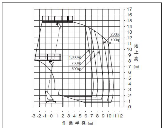
AT150S作業範囲図 アウトリガ最大張出
